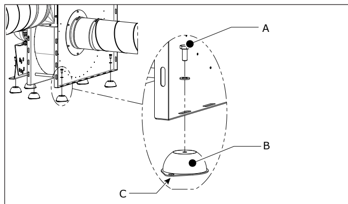
Fig. 4.1 Vibrationsdämpare
