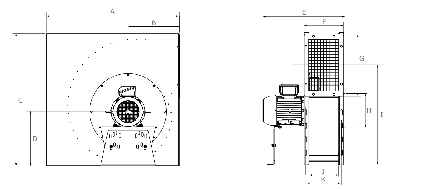
Fig. II Mått TEV
