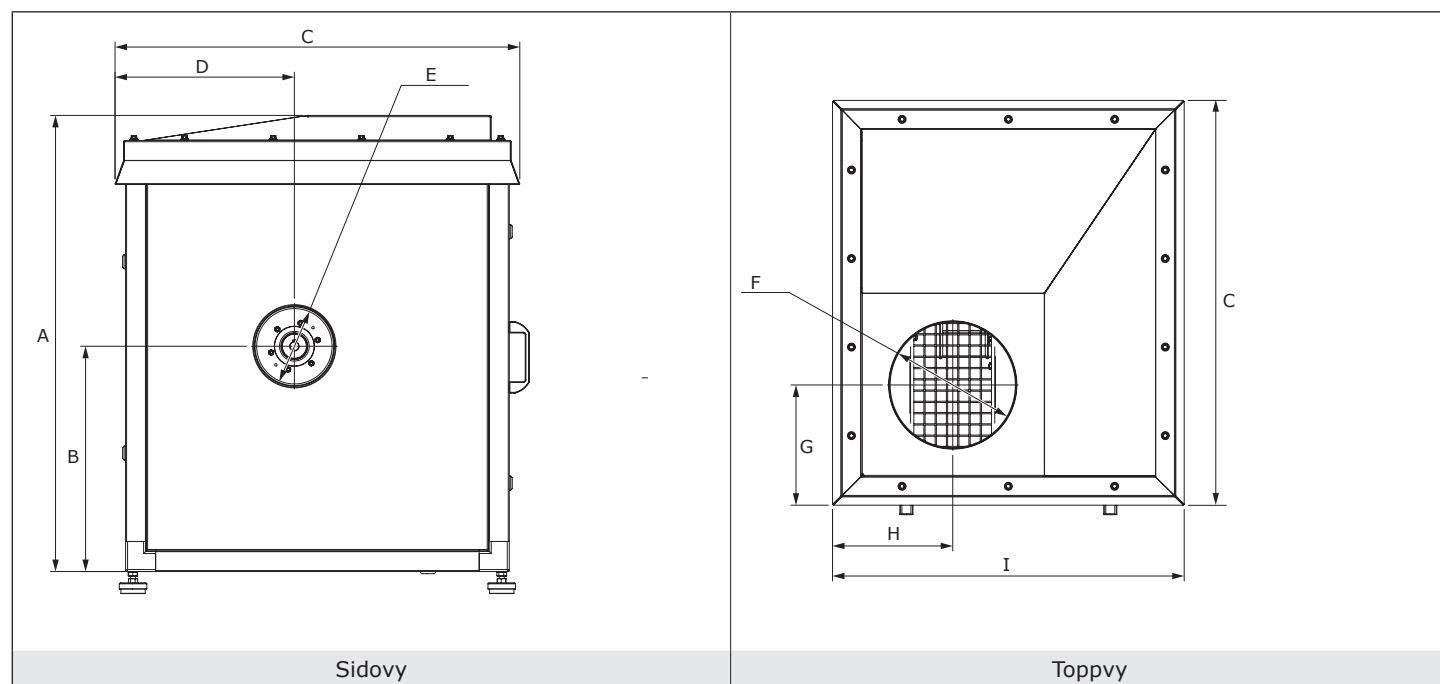
Fig. III Mått SAF
