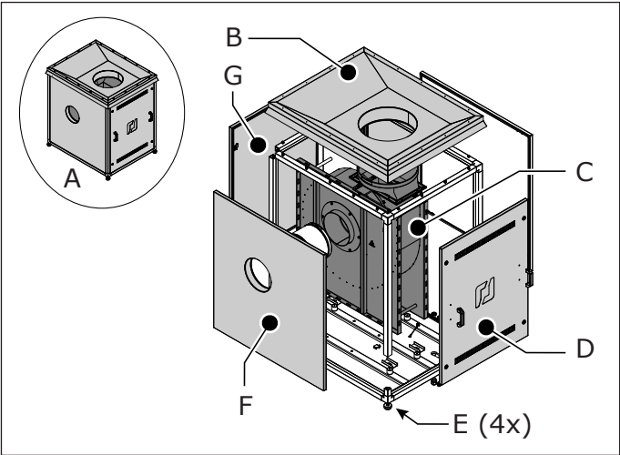
Fig. 2.2 Huvudkomponenter SAF
