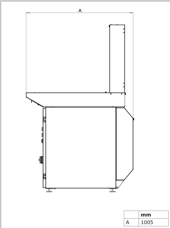
Utsugsbord med bakre utsugspanel (vy från sidan)
