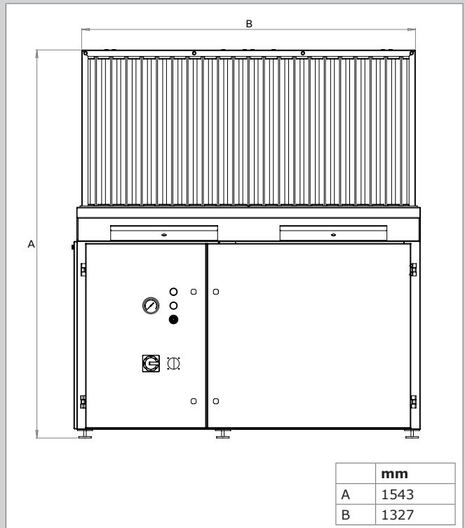
Utsugsbord med bakre utsugspanel (vy framifrån)
