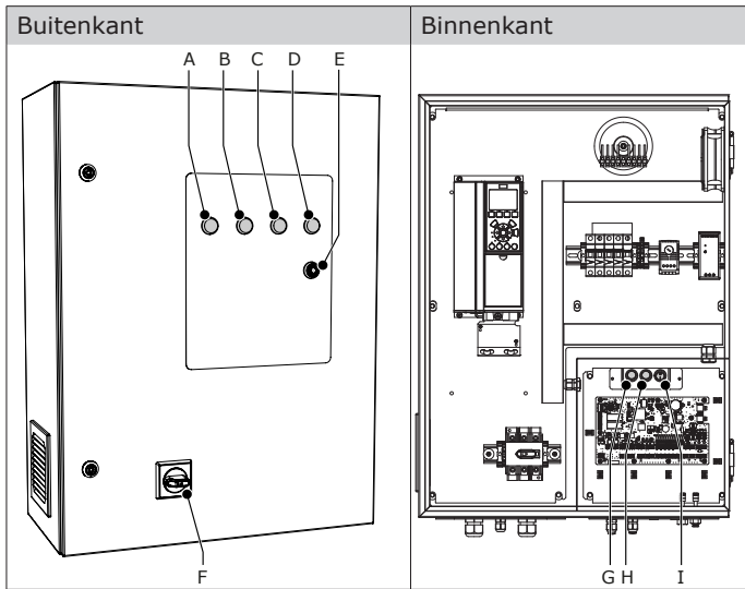
Fig. 6.1 Bedieningspaneel
