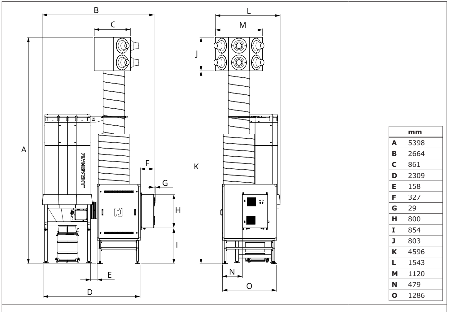
Fig. I Afmetingen SCS-Diluter
