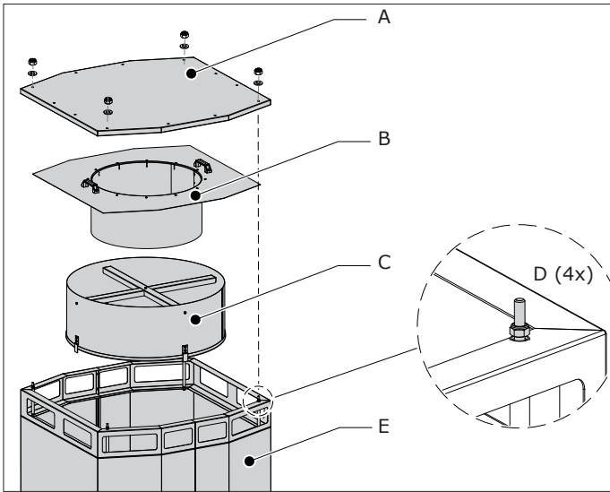
Fig. 4.3 Labyrint vonkenvanger
