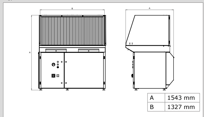
Afzuigtafel met kit voor achterafzuiging en zijpanelen (vooraanzicht)
