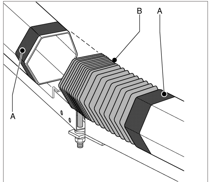
Fig. 4.4 Tubo flessibile intermedio
