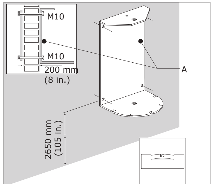
Fig. 4.1 Montage der Wandkonsole
