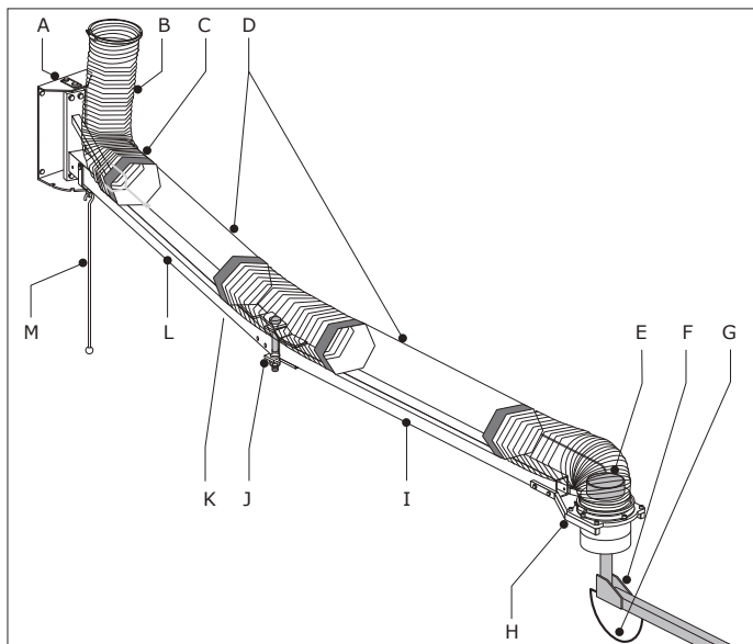
Fig. 2.1 Hoofdc componenten en -elementen
