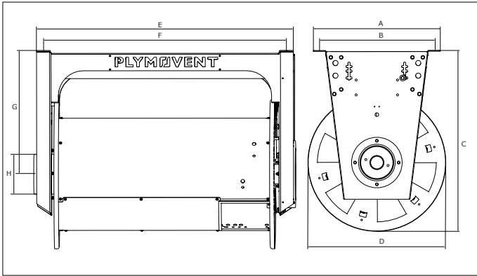
Fig. 4.9 SER dimensions
